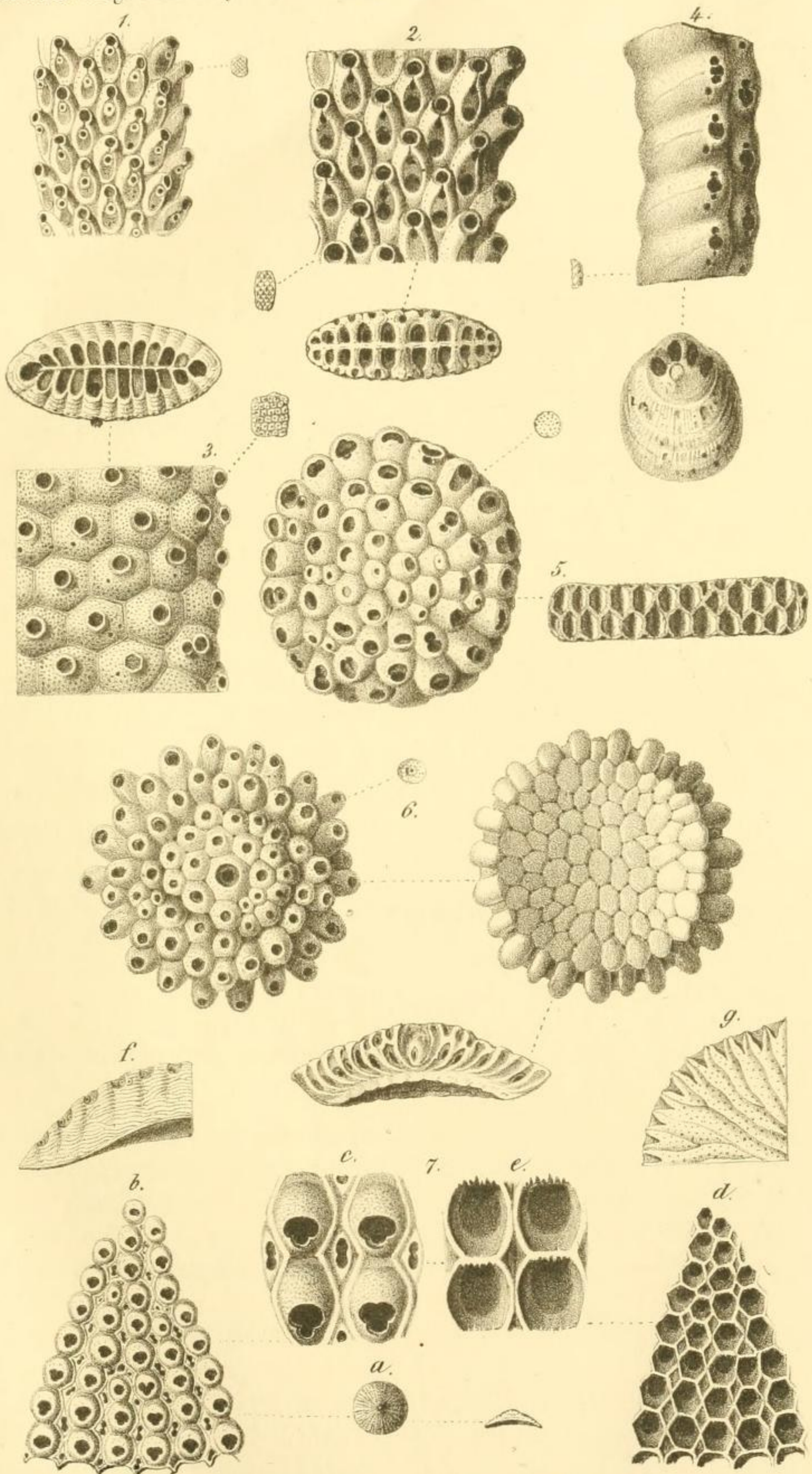
Fig. 5. Orbitulipora Haidingeri Stol.
